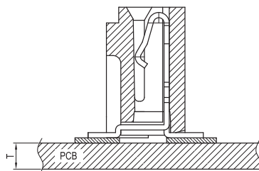
PCB ASS'Y
