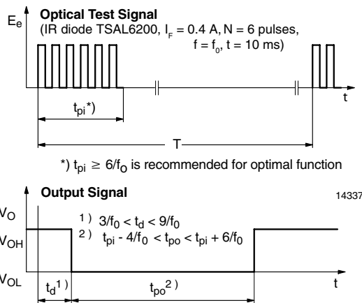
Fig. 1 - Output Function
