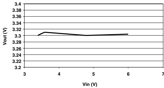
Vout Vs. Vin* Iout = 0.1A
