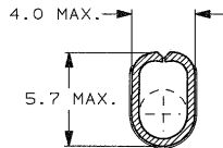
SEZIONE A-A SECTION A-A
