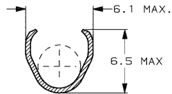
SEZIONE B-B SECTION B-B
