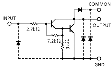
TD62003APG/AFG
