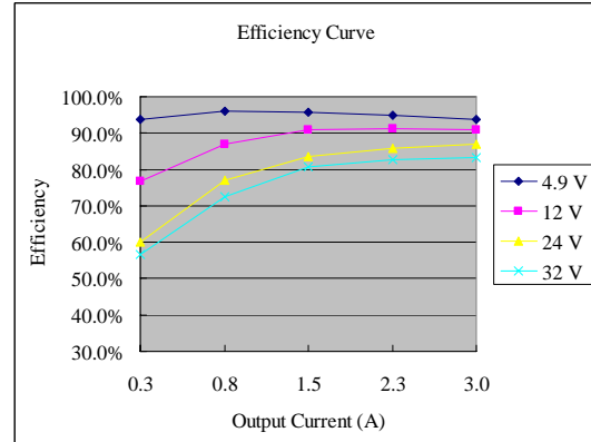
Vo=3.3 V
