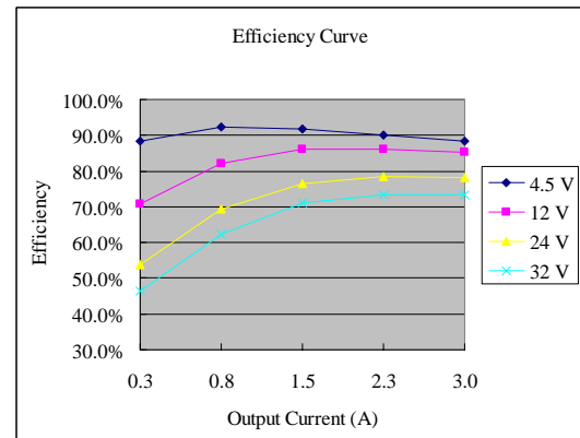
Vo=1.8 V
