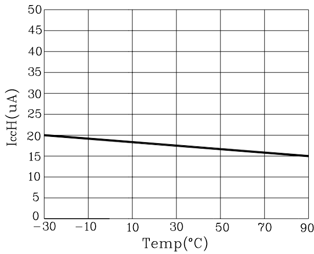
Fig. 3 I_{CCH} - Temp
