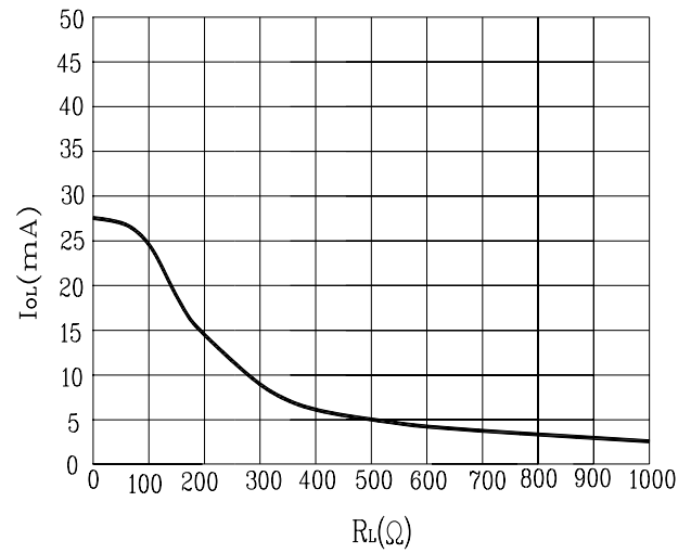
Fig. 4 I_{OL} - R_L
