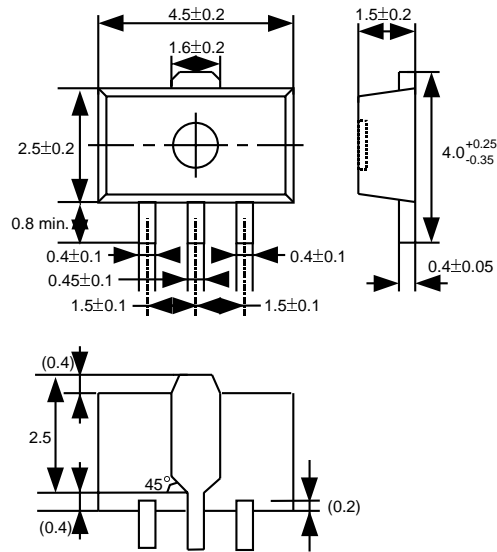
(2) SOT-89-3
