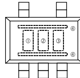
(3) SOT-23-5
