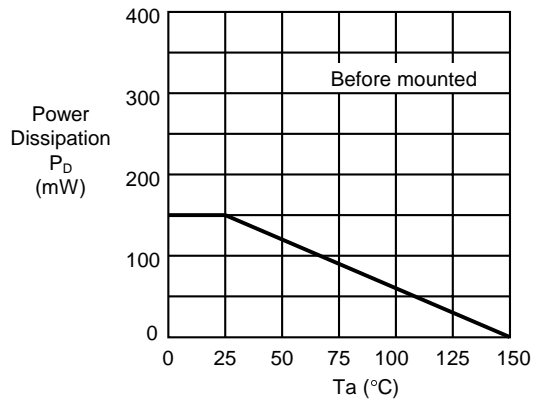
(3) SOT-23-5
