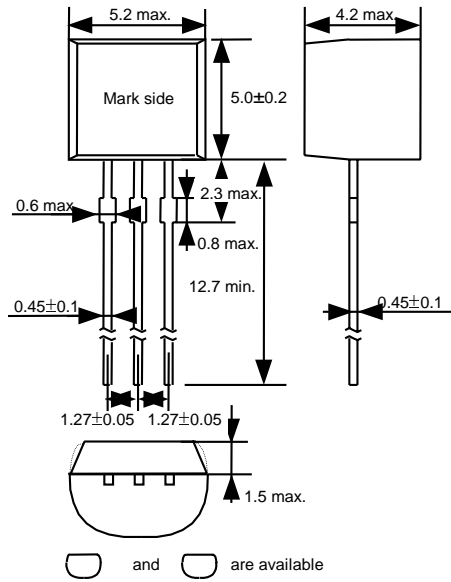
(1) TO-92
