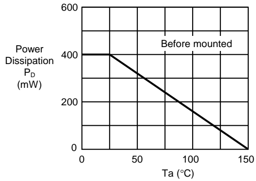
(1) TO-92
