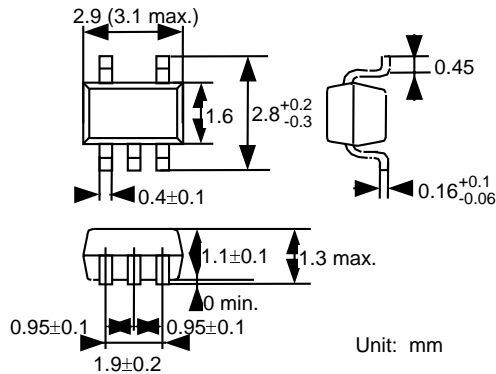
(3) SOT-23-5
