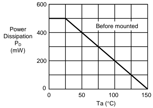
(2) SOT-89-3
