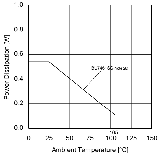
(d) BU7461SG
