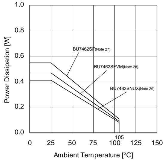
(f) BU7462Sxxx
