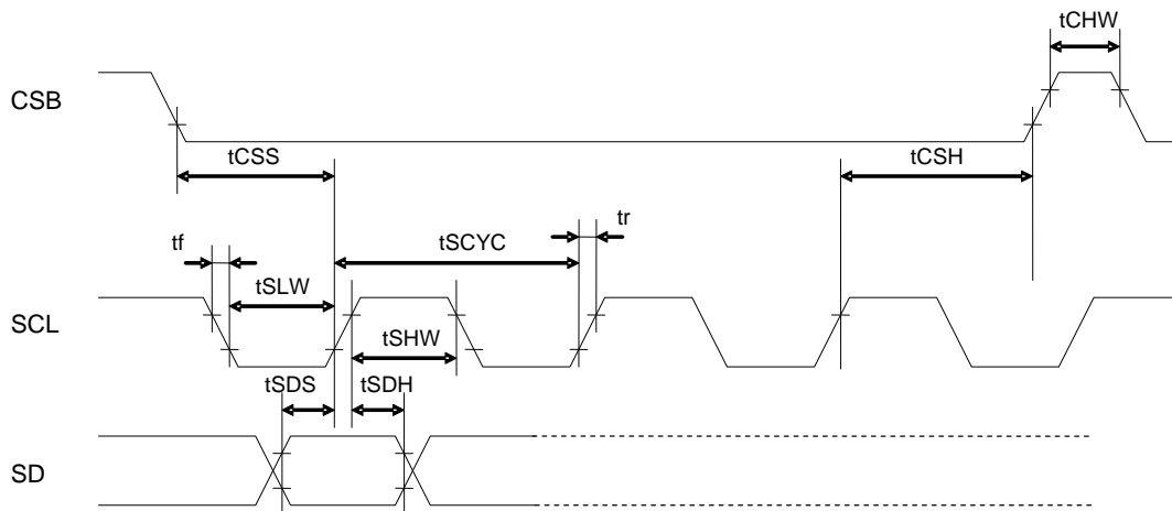
Fig.2 Interface Timing (BU9794AKV)
