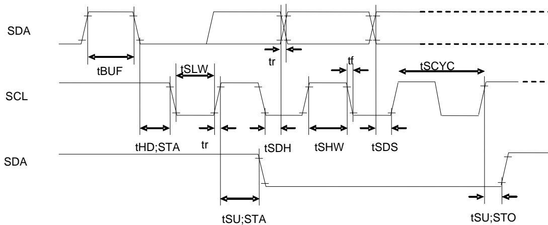
Fig.3 interface timing (BU97950FUV)
