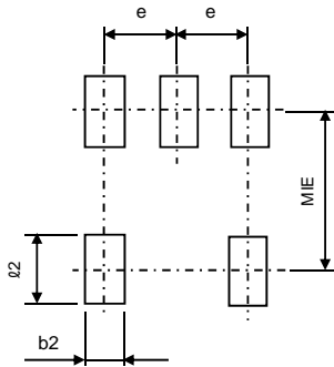
SSOP5
