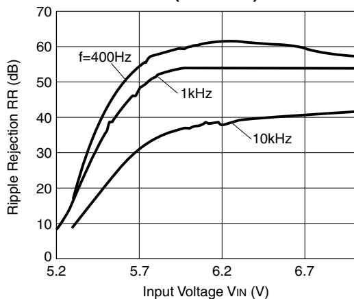
R5510H (VR=5.0V)
