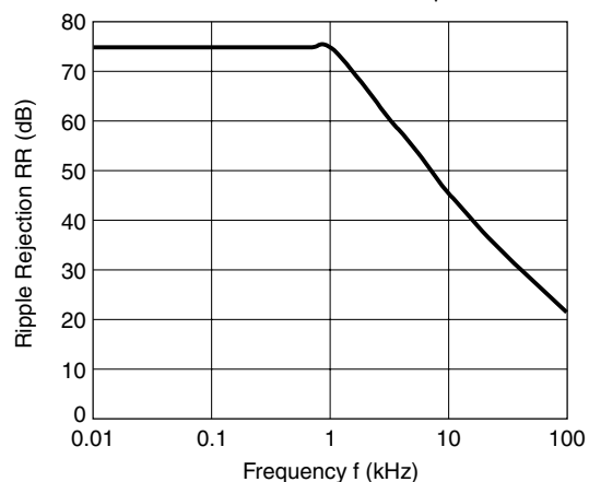
R5510H (VR=4.5V)
