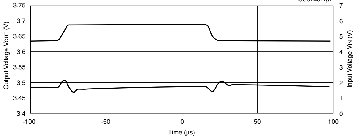
R5510H (VR=3.5V)
