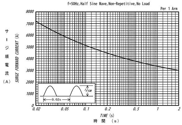
サージ順電流定格 SURGE CURRENT RATINGS
