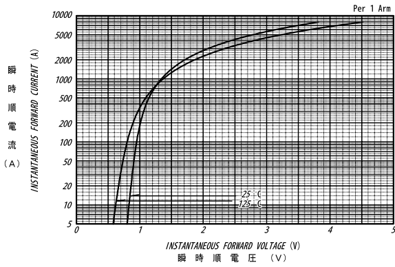
順電圧特性 FORWARD CURRENT VS. VOLTAGE
