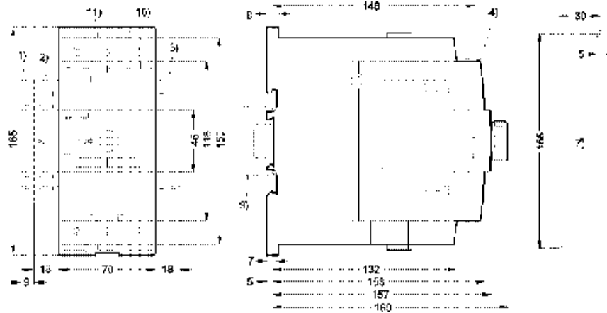
Circuit-breaker J7MN-100
