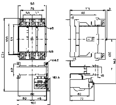
J7KN-200 + J7TKN-210
