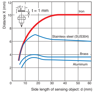
E2E-CR8
