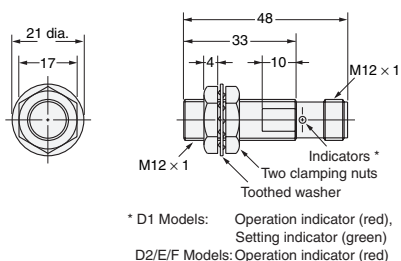
Diagram 22 E2E-X2Y□-M1
