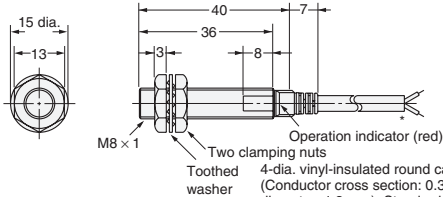
Diagram 7 E2E-X1R5Y□
