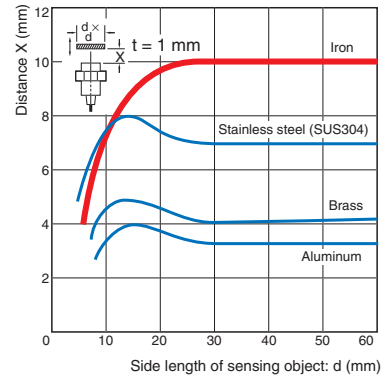
E2E-X10ME/-X10MY/-X10MF
