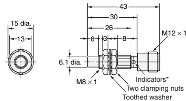
Diagram 19 E2E-X4MD□-M1(G) E2E-X2ME□-M1/E2E-X2MF□-M1
