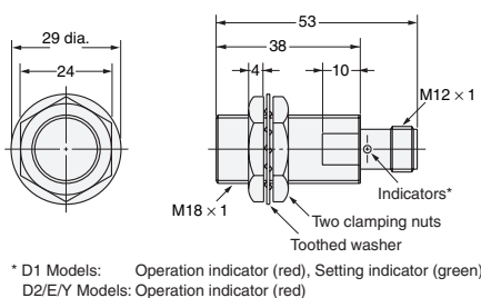
Diagram 26 E2E-X10D□-M1(G)/E2E-X10E□-M1/X10F□-M1 E2E-X10Y□-M1
