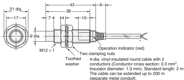
Diagram 12 E2E-X5MY□
