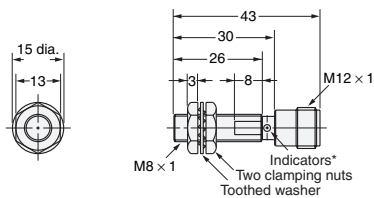
Diagram 18 E2E-X2D□-M1(G) E2E-X1R5E□-M1/E2E-X1R5F□-M1
