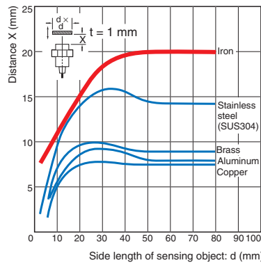
E2E-X5E/-X5Y/-X5F
