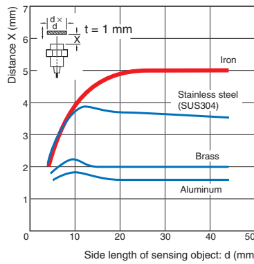
E2E-CR6
