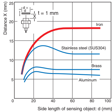
E2E-X18ME/-X18MY/-X18MF
