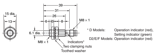
Diagram 29 E2E-X4MD□-M3G/E2E-X2ME□-M3/X2MF□-M3
