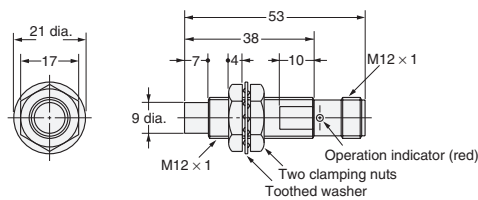
Diagram 25 E2E-X14MD□-M1(G)/E2E-X10ME□-M1 X10MF□-M1 E2E-X10MY□-M1
