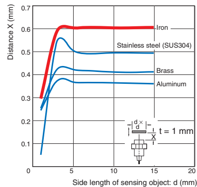
E2E-CR6
