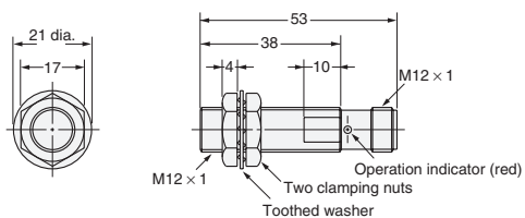
Diagram 24 E2E-X7D□-M1(G)/E2E-X5E□-M1/X5F□-M1 E2E-X5Y□-M1
