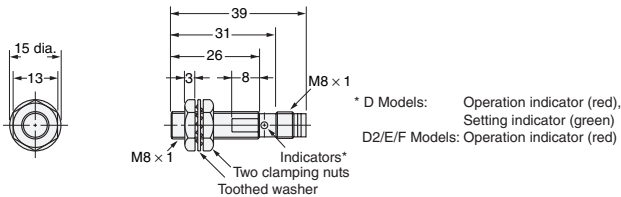
Diagram 28 E2E-X2D□-M3G/E2E-X1R5E□-M3/X1R□-M3
