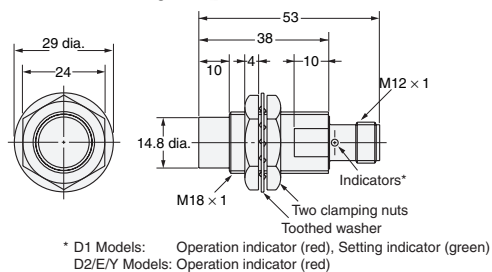
Diagram 27 E2E-X20MD□-M1(G)/E2E-X18ME□-M1/ X18MF□-M1 E2E-X18MY□-M1
