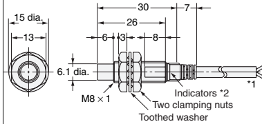
Diagram 6 E2E-X4MD□ E2E-X2ME□/F□
