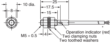
Diagram 4 E2E-X1B□/X1C□
