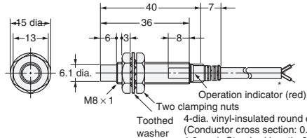
Diagram 8 E2E-X2MY□
