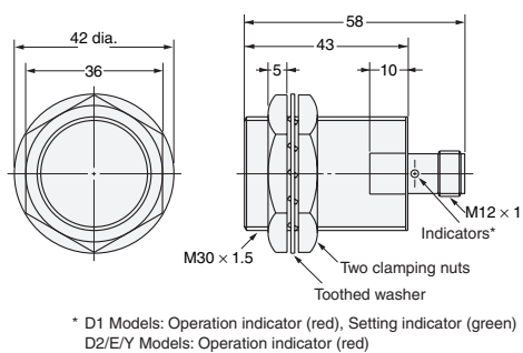
Diagram 26 E2E-X10D□-M1(G)/E2E-X10E□-M1/X10F□-M1 E2E-X10Y□-M1
