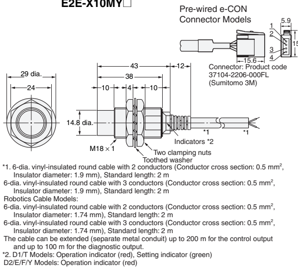
Diagram 15 E2E-X14MD□/E2E-X10ME□/F□ E2E-X10MY□
