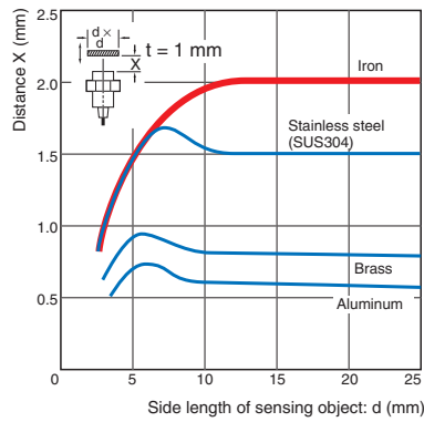
E2E-X2ME/-X2MY/-X2MF
