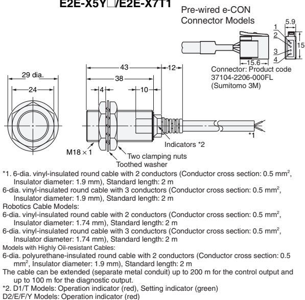
Diagram 14 E2E-X7D□/E2E-X5E□/F□ E2E-X5Y□/E2E-X7T1
