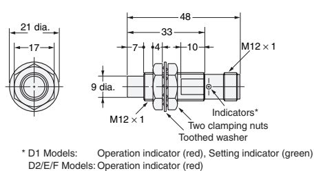
Diagram 23 E2E-X5MY□-M1
