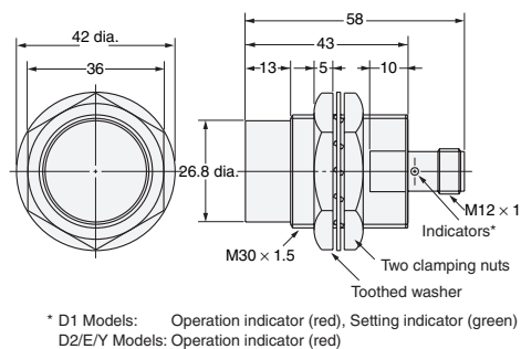
Diagram 27 E2E-X20MD□-M1(G)/E2E-X18ME□-M1/ X18MF□-M1 E2E-X18MY□-M1
