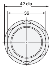
Diagram 35 E2E-X10D□-M1GJ E2E-X10D□-M1J-T E2E-X10D□-M1TGJ-U *3 E2E-X10D1-M1TGJ
