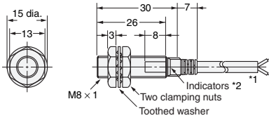
Diagram 5 E2E-X2D□ E2E-X1R5E□/F□
