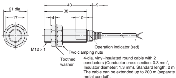
Diagram 11 E2E-X2Y□
