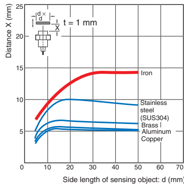
E2E-X2E/-X2Y/-X2F
