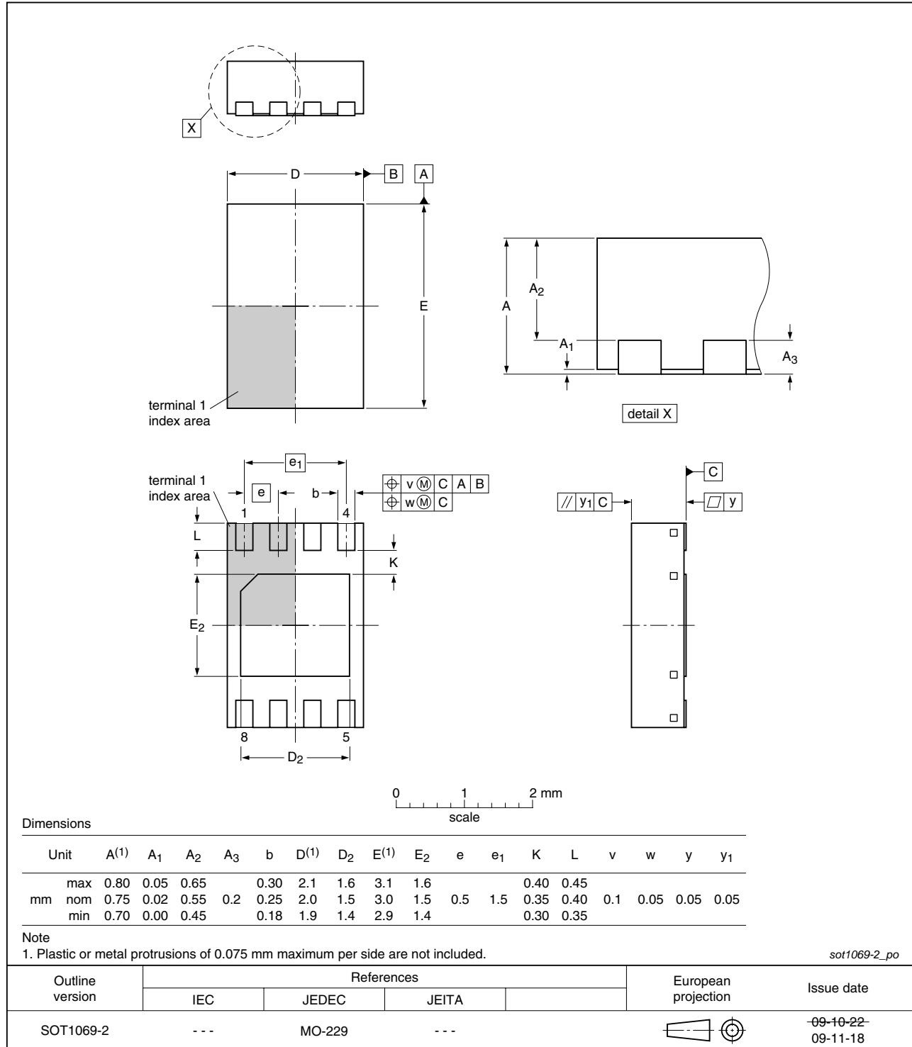
Fig 29. Package outline SOT1069-2 (HWSO88)
