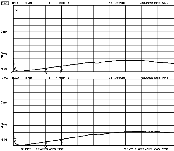
VSWR (f=10MHz~3GHz)
