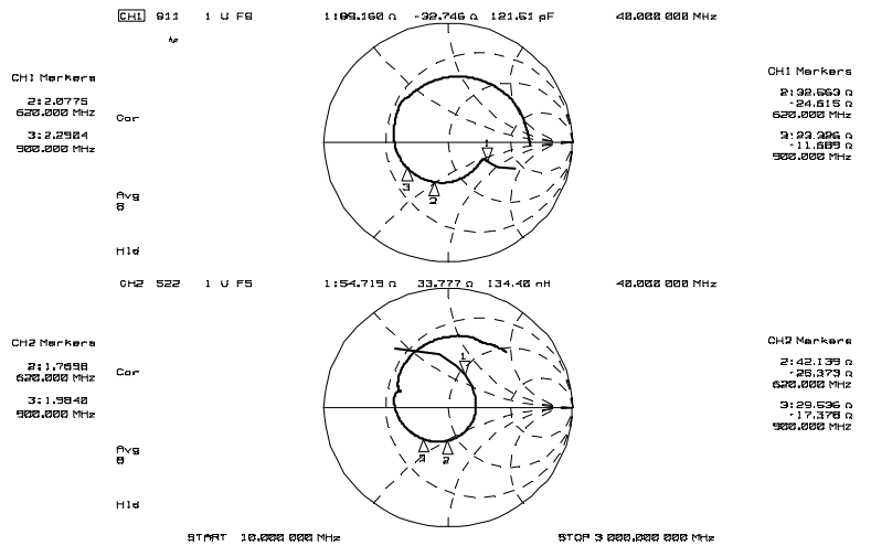
Zin, Zout (f=10MHz~3GHz)
