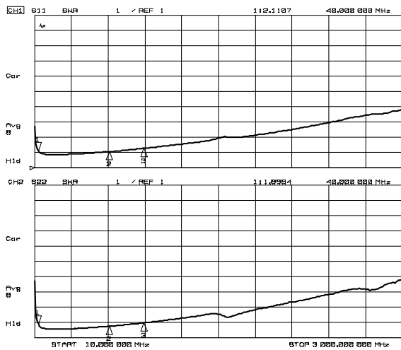
VSWR (f=10MHz~3GHz)
