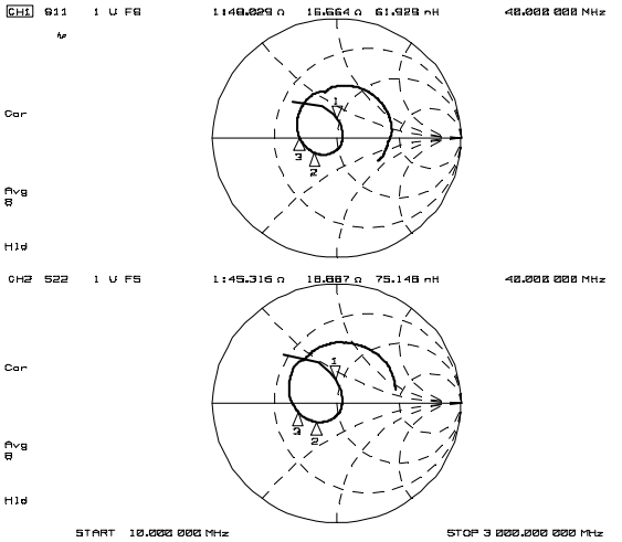
Zin, Zout (f=10MHz~3GHz)
