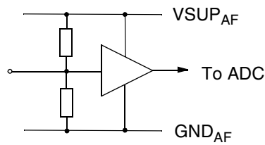
Fig. 6-10: Input pins CIN1, CIN2
