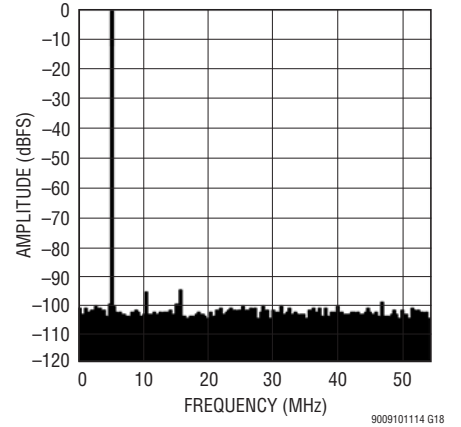
LTM9010-14: 8k Point FFT, f_{IN} = 5\text{MHz} , -1\text{dBFS} , 105\text{Mpsps}
