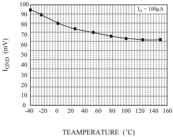
Fig. 9 I_{GND} - TEMP
