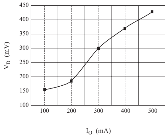
Fig. 3 V_D - I_{OUT}
