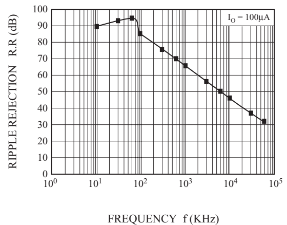
Fig. 6 f - R.R
