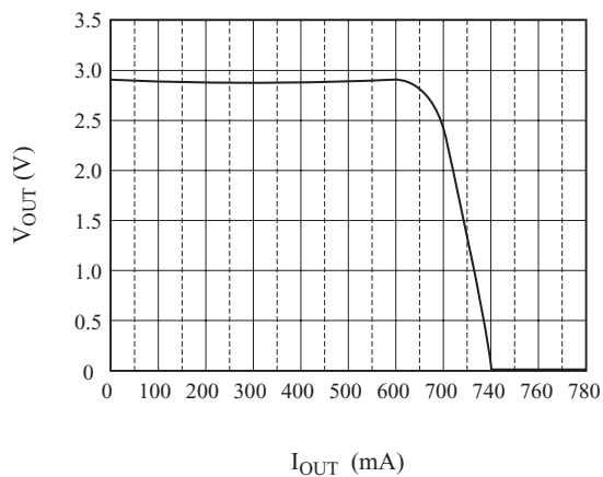
Fig. 5 V_{OUT} - I_{OUT}
