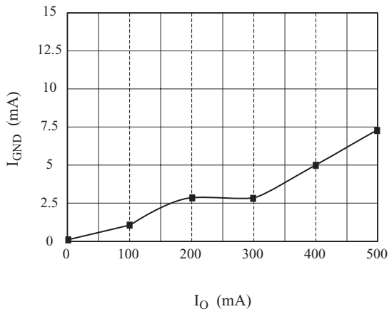
Fig. 1 I_{GND} - I_O
