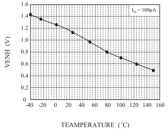
Fig. 8 V_{ENH} - TEMP
