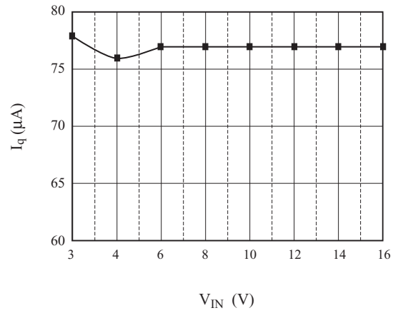
Fig. 2 I_q - V_{IN}
