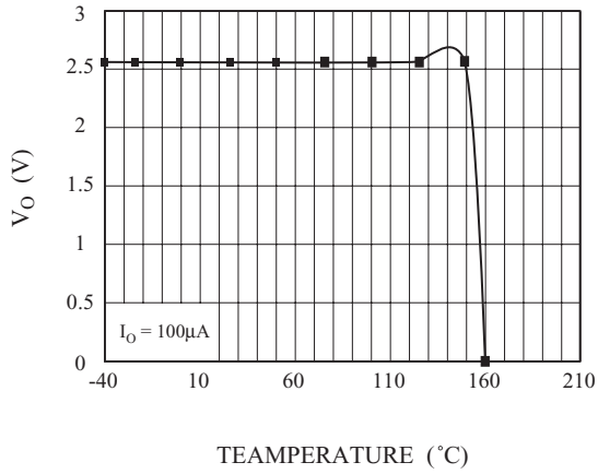
Fig. 7 V_{OUT} - TEMP
