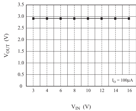
Fig. 4 V_{OUT} - V_{IN}
