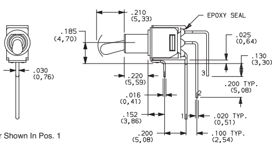
Actuator Shown In Pos. 1
