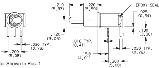
Actuator Shown In Pos. 1
