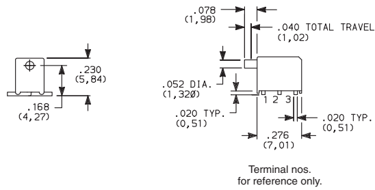
GP12MSCBE SPDT
