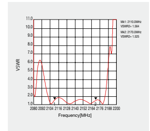
VSWR(OUTPUT)
