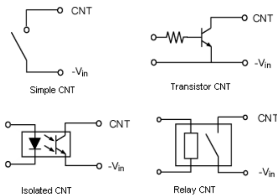
Fig. 51 CNT Circuit
