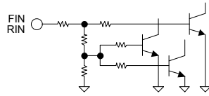
Fig. 38 FIN, RIN
