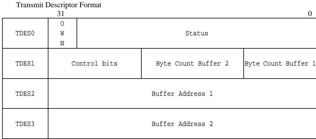
Fig - 6 Transmit Descriptor Format
