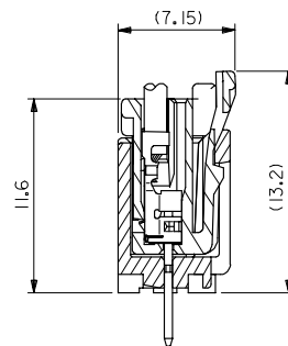
嵌合断面図
