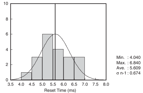
b) Reset time
