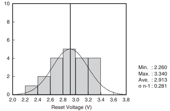
b) Reset voltage
